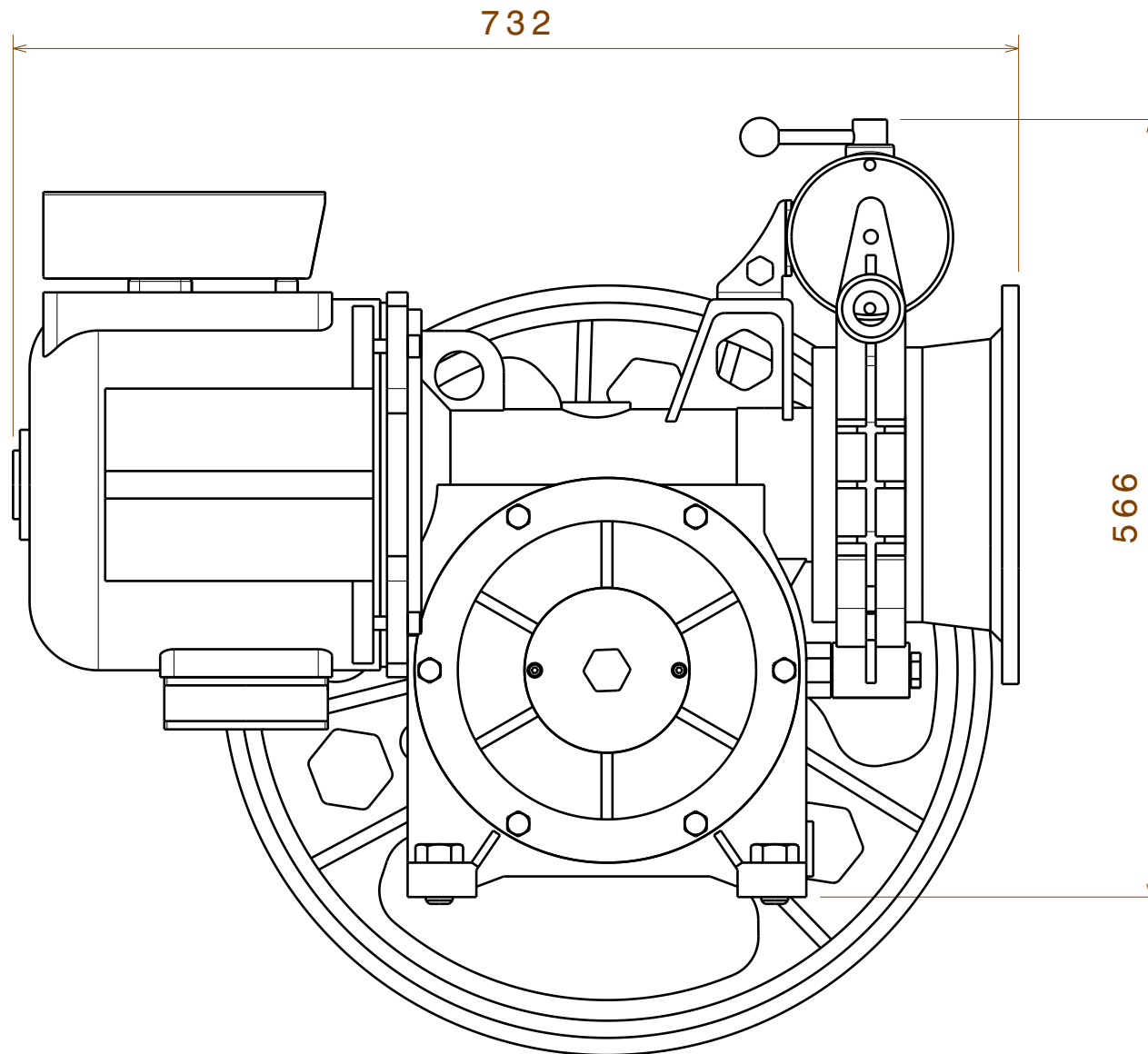
Front view Scale: 1:5
