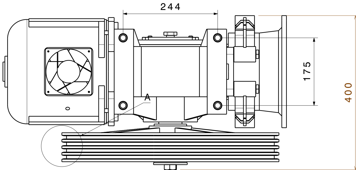
Front view Scale: 1:5
